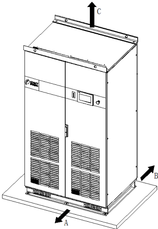
图 3-4 安装空间距离示意图
