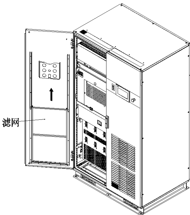
图 4-4 滤网更换示意图
