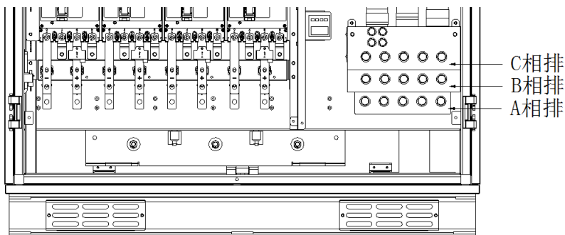
图 3-12 交流输出铜排位置示意图
