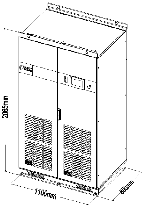
图3-1 外形尺寸示意图
