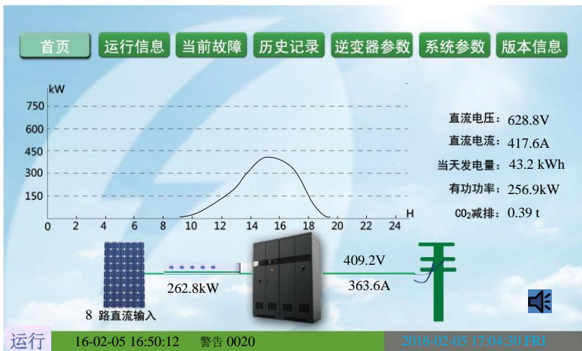
图 5-2 首页界面
