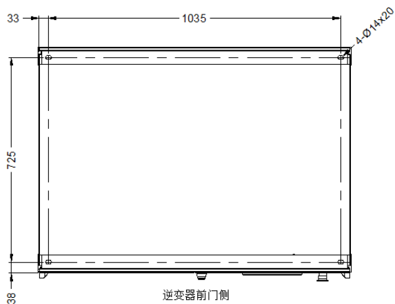
图 3-3 安装固定孔尺寸图
