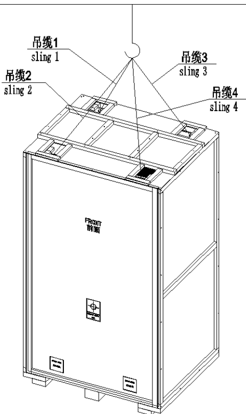
图 3-5 吊车搬运示意图
