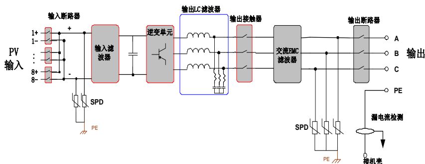
图 2-2 CPS SCA630/500KTL-H/CN 原理框图
