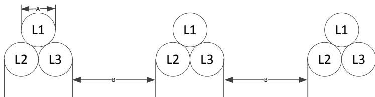
图3-16 交流侧线缆沟布局
