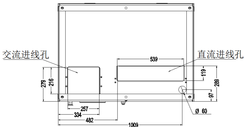
图 3-2 进出线孔位置尺寸图
