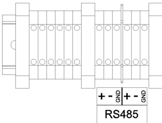
图3-18 RS485通讯连接端子图
