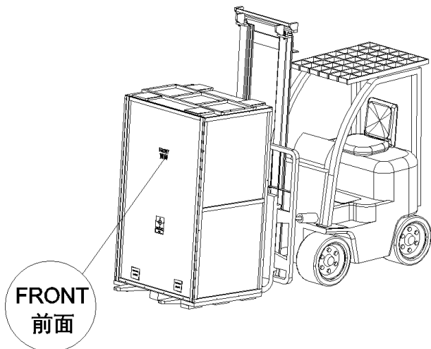
图 3-6 叉车搬运示意图
